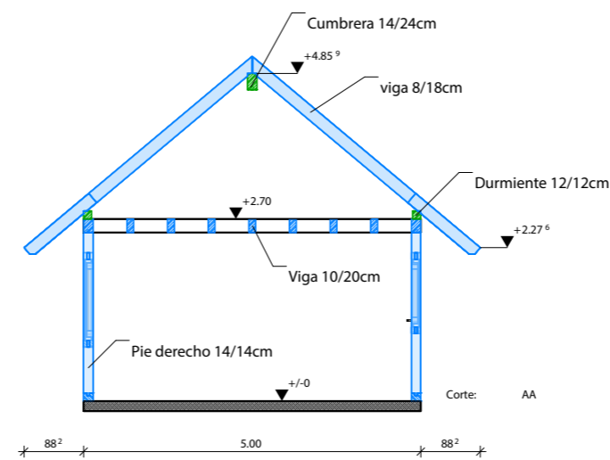
Corte A-A
